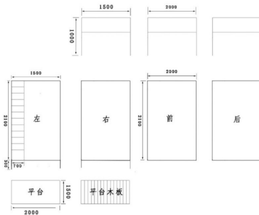
图 20：裁判台施工图纸
